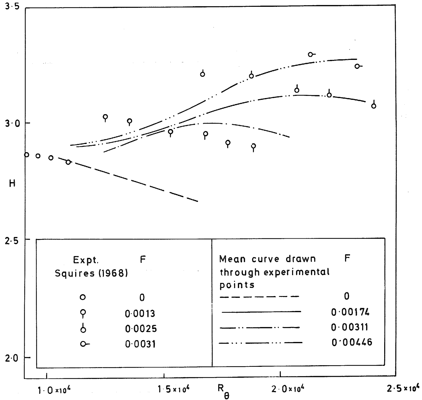
FIG. 27. H vs R_\theta ( M=1.8 ).
