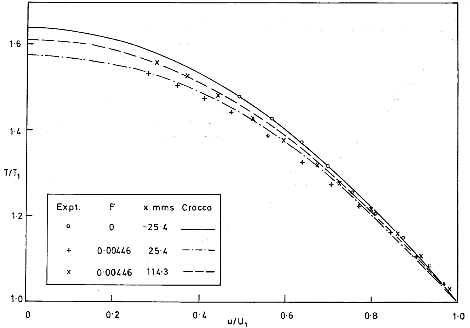
FIG. 22. T/T_1 vs u/U_1 ( M=1.8 ).
