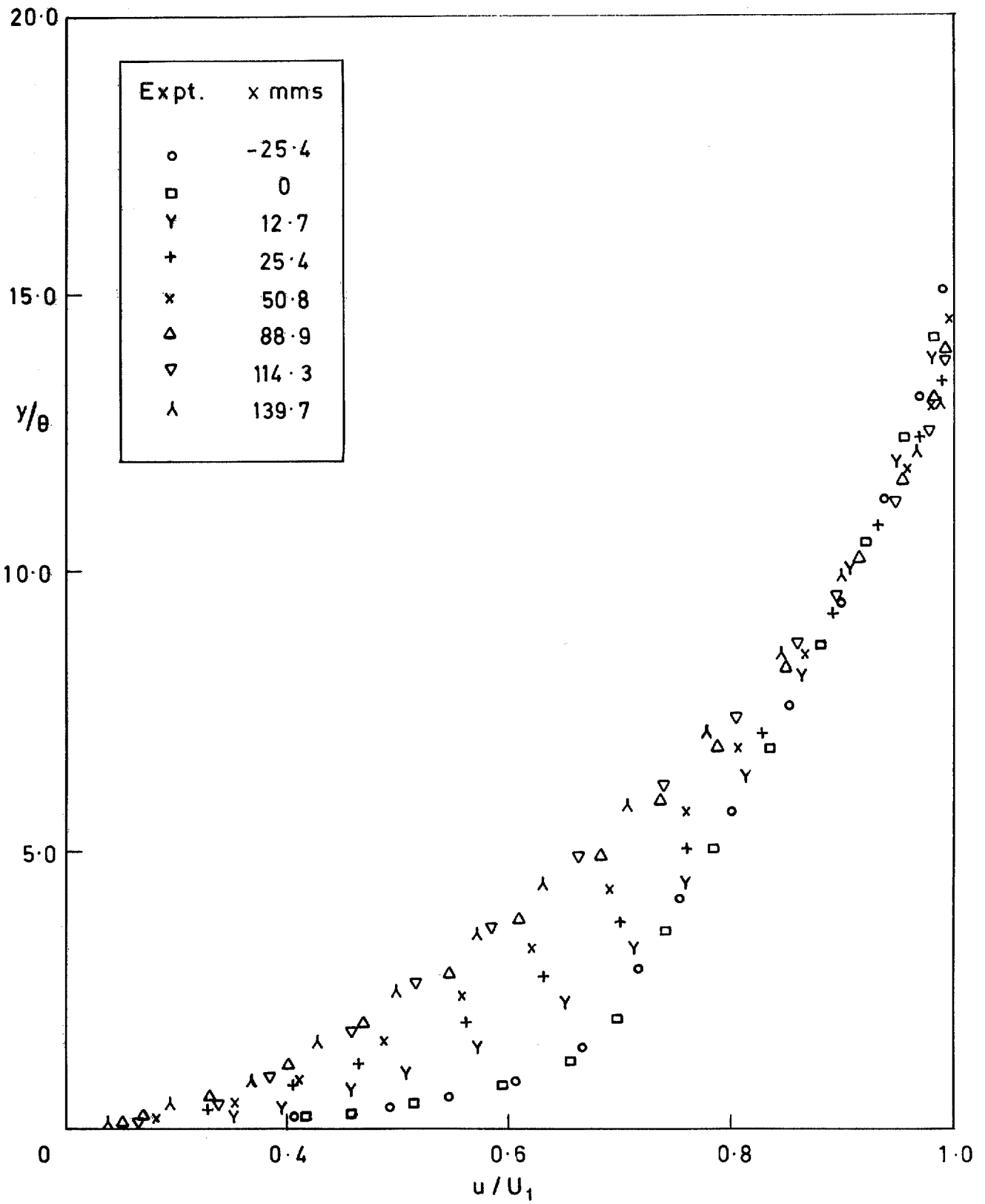
FIG. 30. y/\theta vs u/U_1 ( M=3.6 ; F=0.00294 ).
