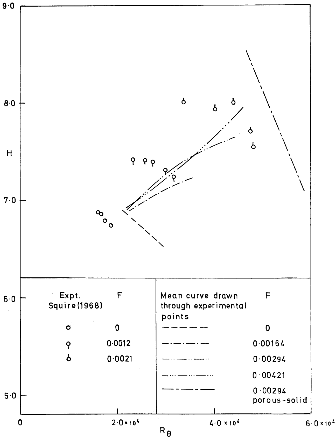
FIG. 28. H vs R_\theta ( M=3.6 ).
