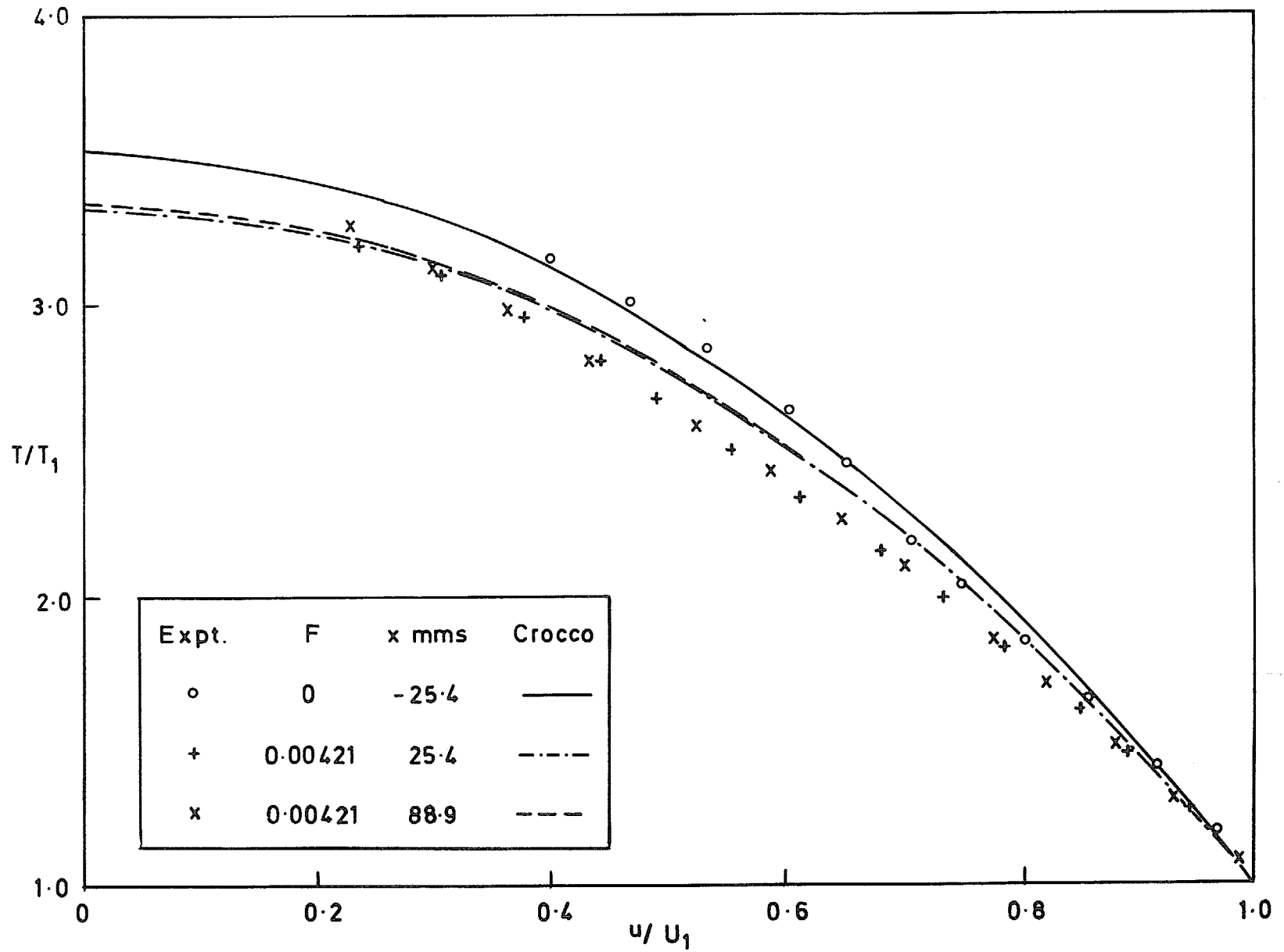
FIG. 23. T/T_1 vs u/U_1 ( M = 3.6 ).
