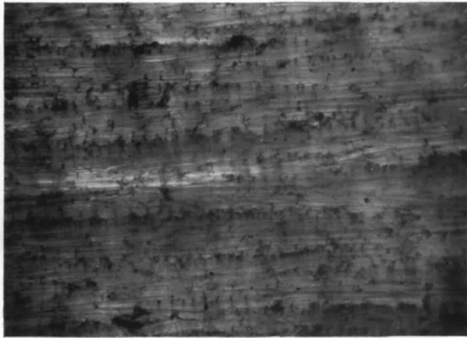
FIG. 6a. No. 2 Balsa. Longitudinal section.
