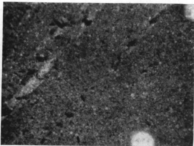
FIG. 9a. No. 7 U.F. Gel. Longitudinal section.
